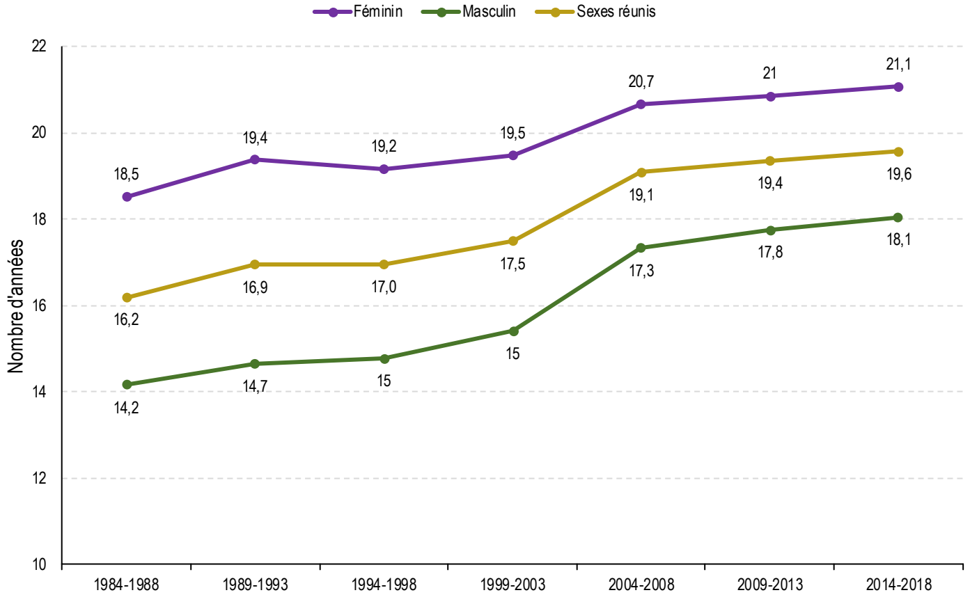
Espérance de vie à 65 ans selon les sexes en Abitibi-Témiscamingue de 1984-1988 à 2014-2018
